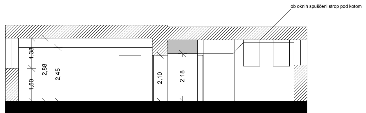
PREREZ B-B
